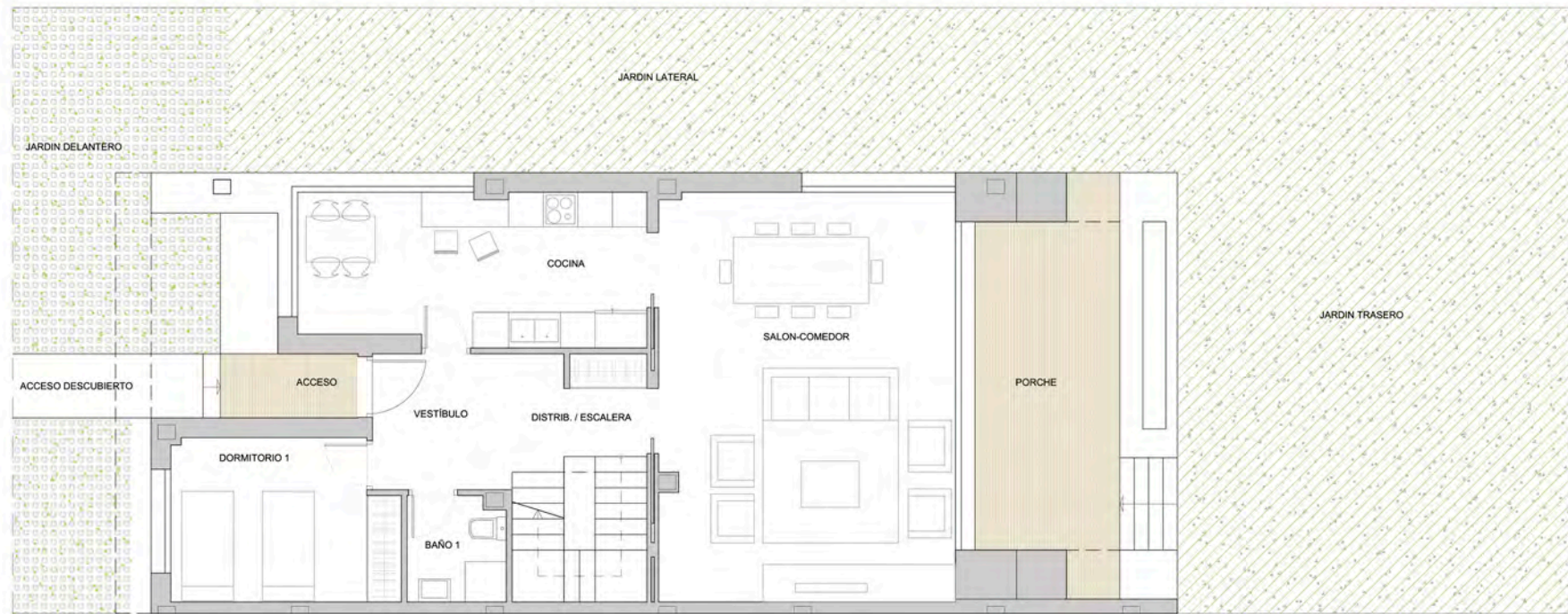
PLANTA BAJA
